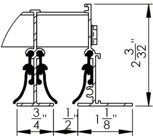
DETALLE B ESCALA 1 : 2
